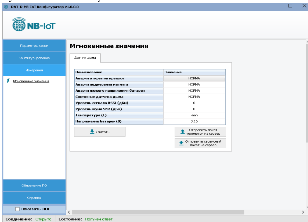
Рисунок 13 — Мгновенные значения
